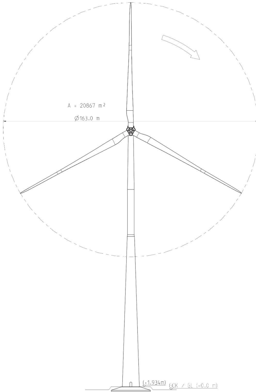
Abbildung 4: Ansicht der Nordex N163/6.X auf 164 m NH, Quelle Fa. Nordex
